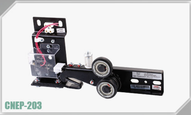
CNEP-203 产品参数 PRODUCT PARAMETERS DOOR LOCKS Left Side Opening the Door Suitable Brand: Mitsubishi, Otis
