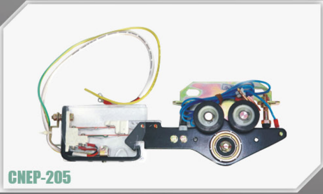
CNEP-205 产品参数 PRODUCT PARAMETERS DOOR LOCKS Side/Center Opening the Door Suitable Brand: Hitachi
